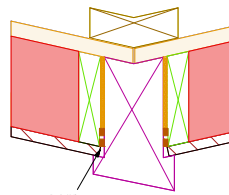
Detail Kehle Mst. 1:10
