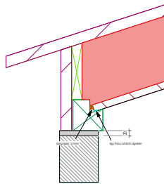
Detail Schwelle Mst. 1:10
